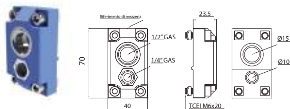
M231-012014 Toma frontal doble Ø25 ½" - Ø16 ¼"
